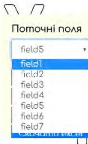
Рисунок 4.4 — Список полів
