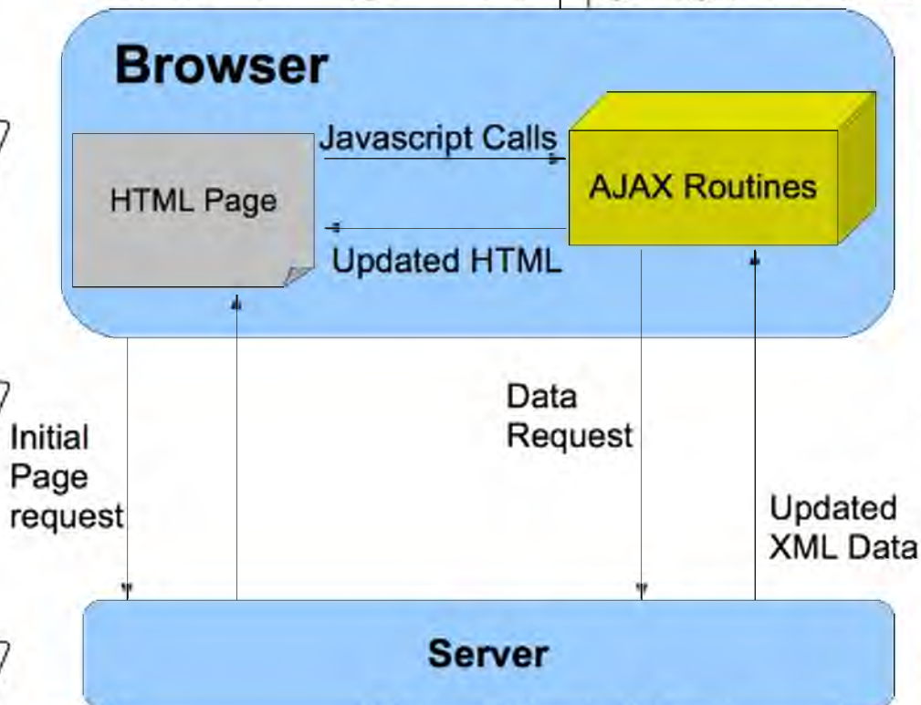
Рисунок 1.2 – Схеми взаємодії HTML-сторінки з сервером засобами AJAX
