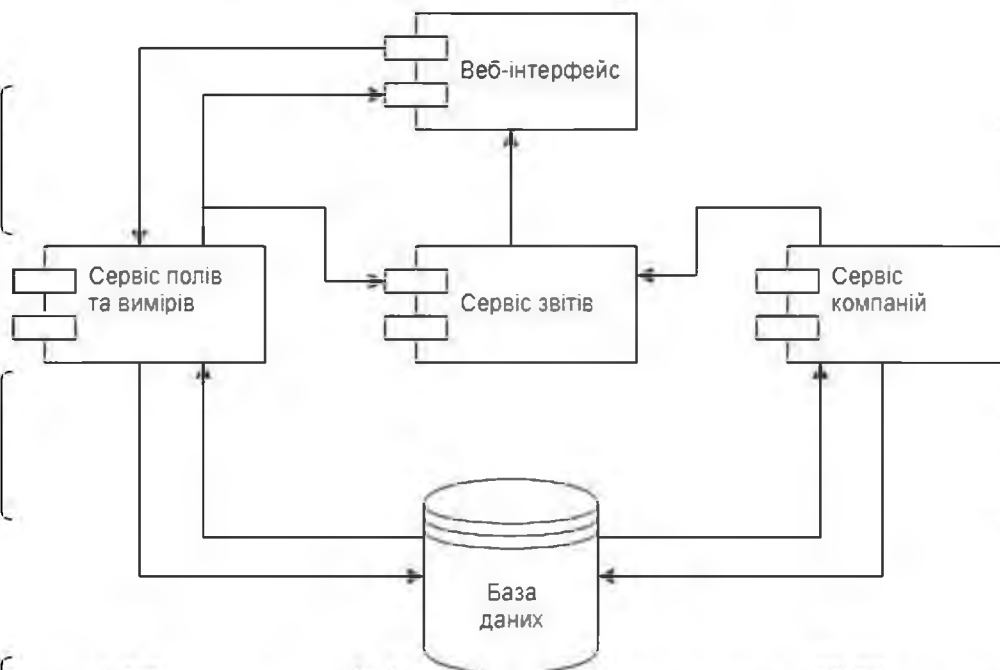
Рисунок 1.1 — Схема взаємодії частини порталу
