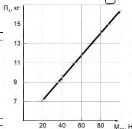
Рис. 2.12. Зміна втрат зерна \Pi_{вз} за підбирачем комбайна залежно від маси M_{оп} опорної поверхні пристрою, що копіює
