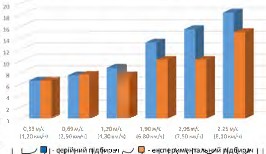
Рис. 4.14. Діаграма втрат зерна за серійною та експериментальною
