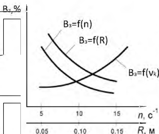
Рис. 2.6. Зміна втрат зерна B_3 за підбирачем комбайна при підборі валків
