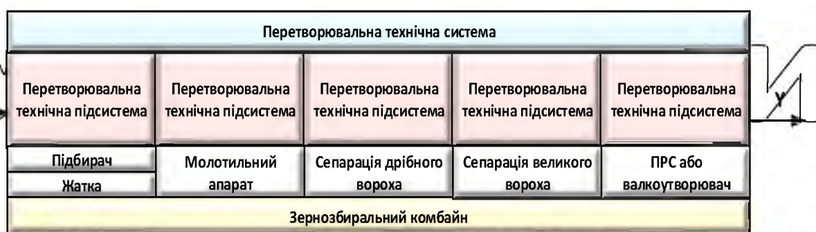
Рис. 2.2 Зернозбиральний комбайн як перетворююча технічна система
