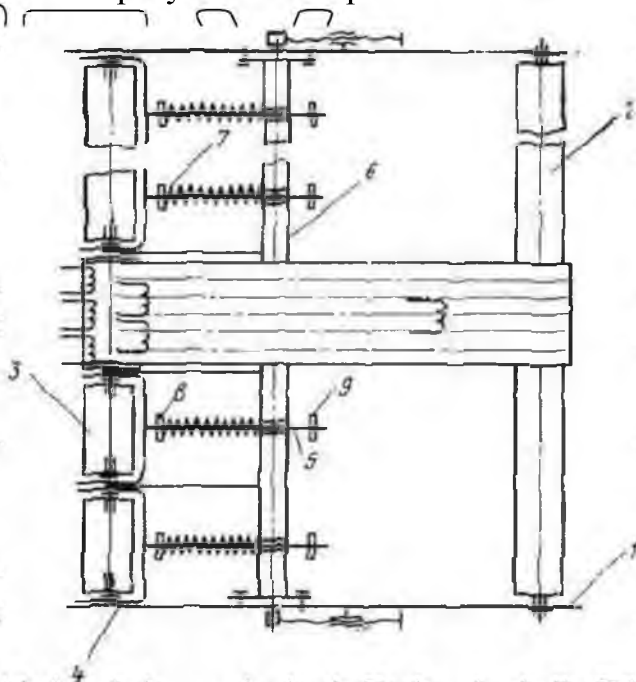
Рис. 1.7. Транспортерний підбирач
