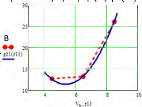
Рис. 4.6. Залежність впливу робочої швидкості руху комбайна TORUM 440 на втрати зерна за платформою-підбирачем
