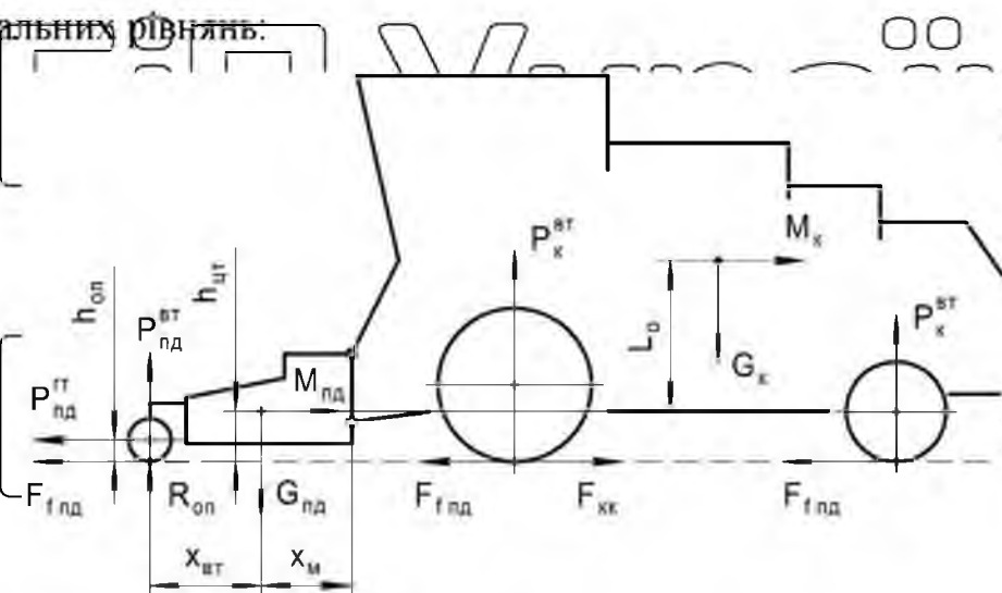
Рис. 2.9. Загальна схема утворення вертикальної сили P_{pd}^{vt} під час руху комбайна з підбирачем при підборі валка хлібної маси
