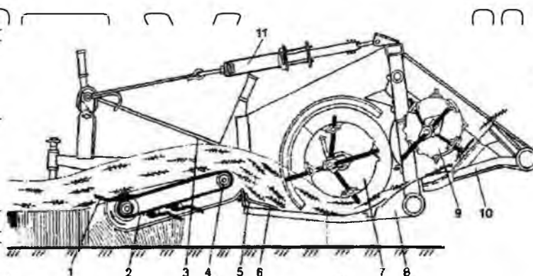
Рис. 1.4. Технологічна схема платформи-підбирача Swa-Pick зернозбирального комбайна TORUM 440
