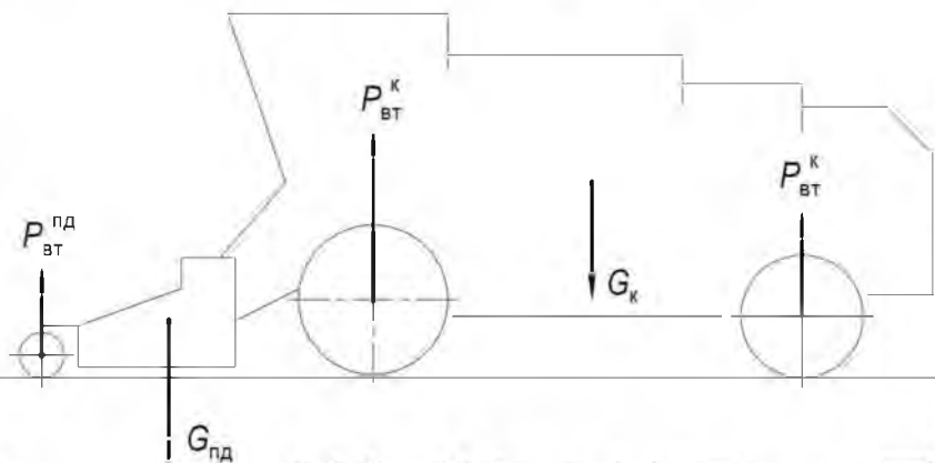
Рис. 2.7. Загальна схема утворення вертикальної сили P_{\text{вт}}^{\text{к}} під час руху зернозбирального комбайна
