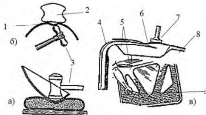
Рис. 16. Деякі прийоми рихтування деталей кузова: а - рихтування
