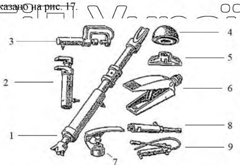
Рис. 17 Гідравлічні пристрої для правки:
