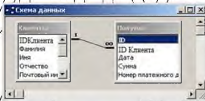
Рис. 1. Схема даних.
